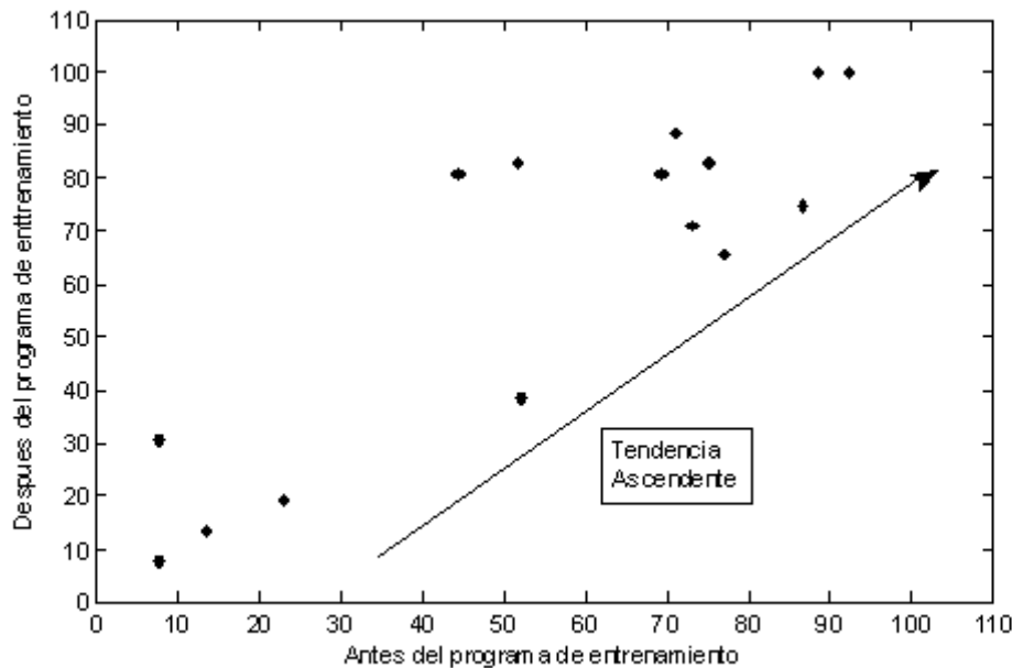
Figura 1. Diagrama de dispersión de los índices del antes y después del programa de entrenamiento en el municipio Mara. Figure 1. Scatter diagram indexes before and after indices of training program in Mara municipality.
