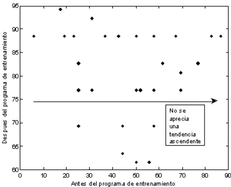
Figura 2. Diagrama de dispersión de los índices del antes y después del programa de entrenamiento en JEL.
