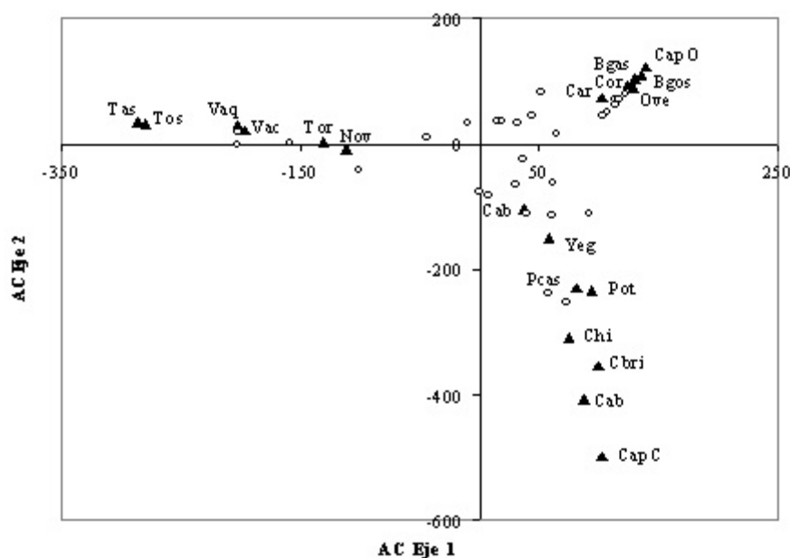
Figura 2: Primeros dos ejes del Análisis de Correspondencia mostrando la posición de las especies y categorías animales (triángulos) y los establecimientos ganaderos (círculos). Tas: terneras. Tos: terneros. Vac: vacas. Vaq: vaquillonas. Nov: novillos. Tor: toros. Bgas: borregas. Bgos: borregos. Cor: corderos. Car: carneros. Ove: ovejas. CapO: capones ovinos. Cab: caballos. Yeg: yeguas. Pcas: potrancas. Ptr: potros. C bri: cabrillas. Chi: chivos. Cab: cabras. CapC: capones caprinos.
