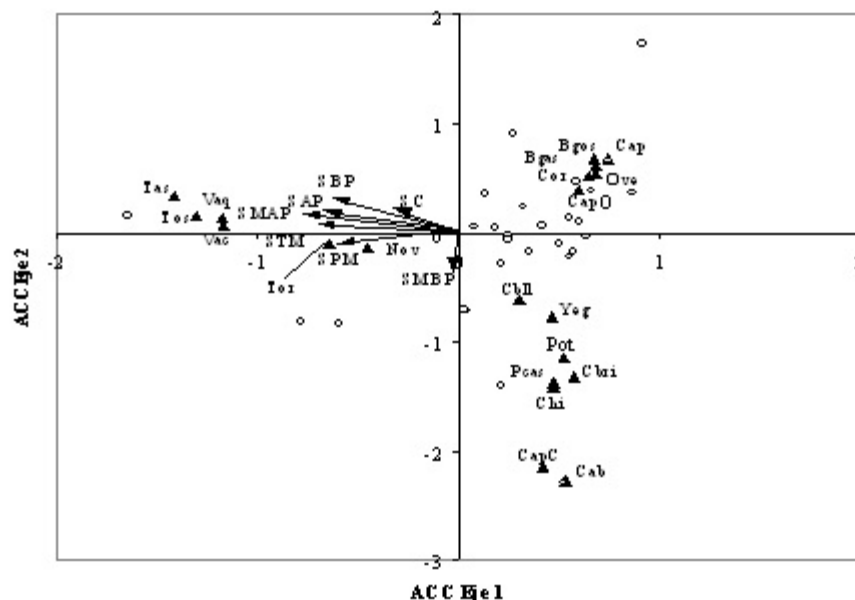
Figura 3: Primeros dos ejes del Análisis de Correspondencia Canónica mostrando la posición de las especies y categorías animales (triángulos), los establecimientos ganaderos (círculos) y las superficies de las distintas clases de mallín y total del establecimiento (vectores). SMAP: superficie mallines de muy alta productividad. SAP: superficie mallines de alta productividad. SPM: superficie de mallines de productividad media. SBP: superficie de mallines de baja productividad. SMBP: superficie de mallines de muy baja productividad. STM: superficie total de mallines. SC: superficie total del establecimiento. Las abreviaturas de las especies y categorías animales son las mismas que en la Figura 2.
