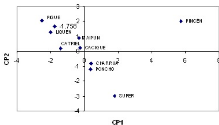
Figura 2: Distribución de los cultivares analizados en el plano de las dos primeras Componentes Principales.
