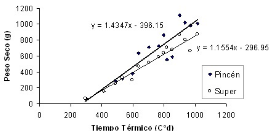
Figura 3: Tasas de crecimiento de las variedades ProINTA Pincén y ProINTA Super. Figure 3: Growth rates of ProINTA Pincen and ProINTA Super varieties.
