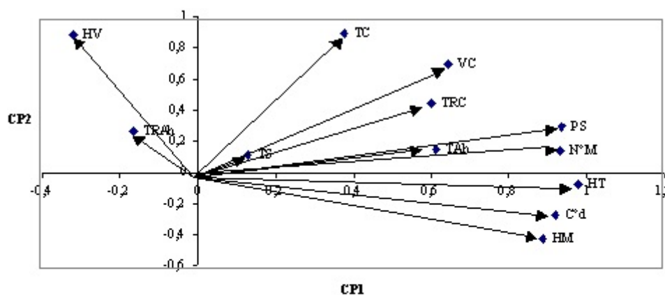
Figura 1: Relación entre las variables utilizadas, representadas en el plano de las dos primeras Componentes Principales.
