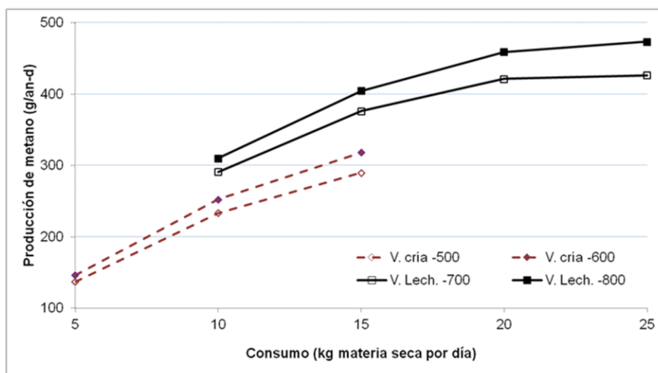
Figura 1. Producción de metano en función del consumo de materia seca en vacas de cría y leche para raciones con digestibilidades entre 500 y 800 g por kg de materia seca.
